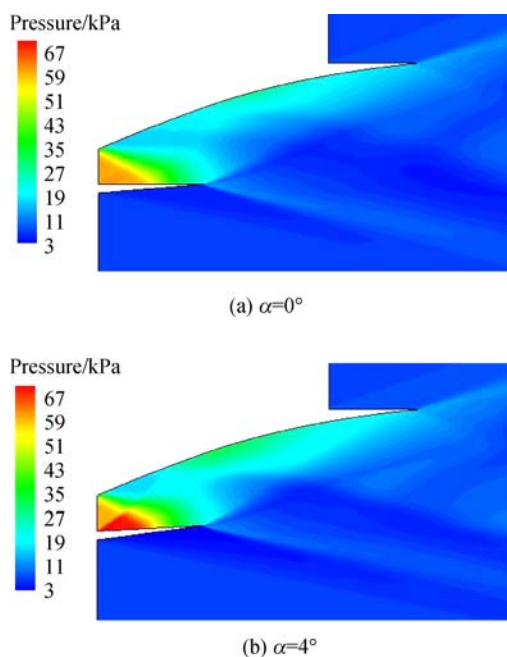
图4 数值模拟不同下唇板角度流场压力云图
