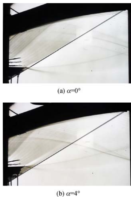
图7 试验纹影照片
