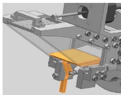
图5 调节机构图
